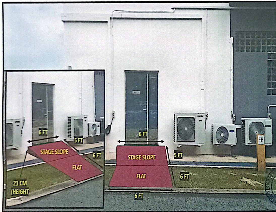
SUKATAN PLATFORM PINTU SEBELAH KIRI BANGUNAN SOKU
