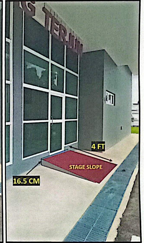
SUKATAN PLATFORM PINTU MASUK BANGUNAN SOKU
