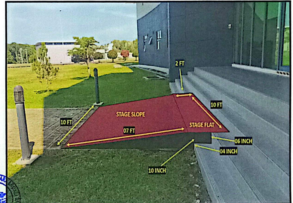
SUKATAN PLATFORM TEMPAT BERGAMBAR BANGUNAN MARKAS RPK ABDB
